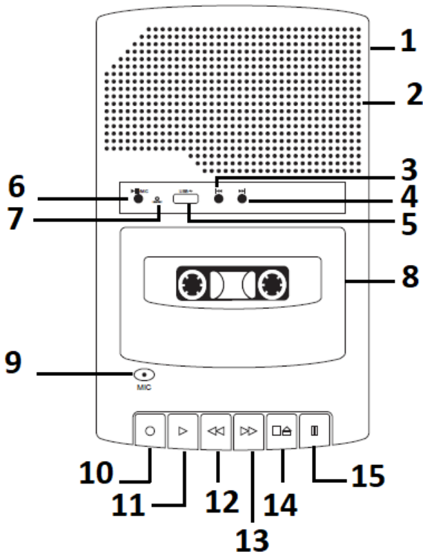
VOORAANZICHT
